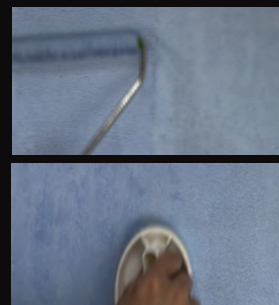
3. 第二道重複第一道工序，將面漆加水20%稀釋攪拌均勻使用滾輪上塗，利用橢圓打磨器進行上下(直紋)或左右(橫紋)打磨，至產生紋路即可待乾燥即完成。
